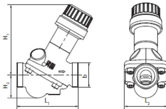
Рис.4 Габаритные и присоединительные размеры.
