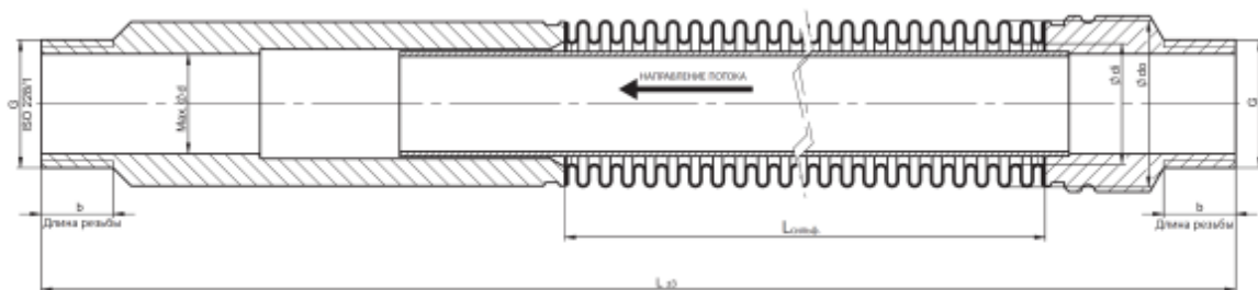
Осевой компенсатор с внутренней гильзой без защитного кожуха
